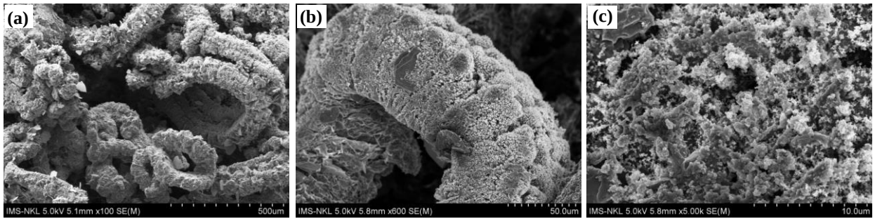
Hình 3.18. Ảnh SEM của mẫu compozit 7n-ZB/7RP/7EG/PP sau thử nghiệm cháy UL94-V ở các độ phóng đại khác nhau
