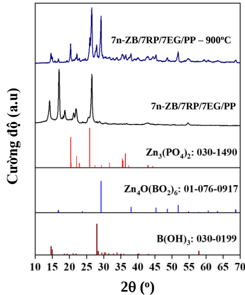
Hình 3.20. Giản đồ XRD của mẫu composit 7n-ZB/7RP/7EG/PP trước và sau khi nung ở 900 °C
