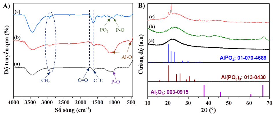
Hình 3.25. Phổ FT-IR (A) và XRD (B) của cặn than các mẫu composit: 10APP@PEI/EP (a), 10ATH PEI /EP (b) và 3ATH PEI /7IFR/EP (c) sau khi nung ở 900 °C
