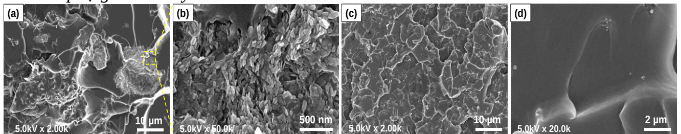
Hình 3.35. Ảnh SEM bề mặt đứt gãy của các mẫu nanocompozit nền nhựa EP sau thử nghiệm kéo: 3HT/7IFR/EP (a, b) và mẫu 3HT 3 /7IFR/EP (c, d)
