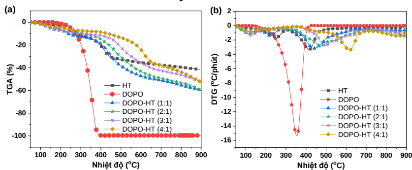
Hình 3.14. Giản đồ TGA (a) và DTG (b) của HT, DOPO và các mẫu DOPO-HT với tỷ lệ DOPO:HT khác nhau trong môi trường khí nitơ (N 2 )
