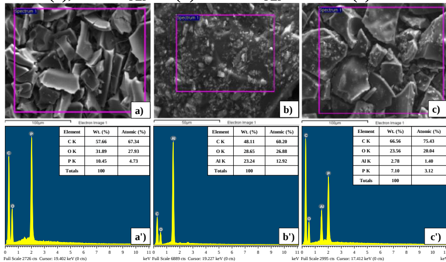
Hình 3.26. Ảnh SEM và giản đồ EDX của cặn than của các mẫu 10APP@PEI/EP (a, a'), 10ATH PEI /EP (b, b') và 3ATH PEI /7IFR/EP (c, c') sau khi nung ở 900 °C
