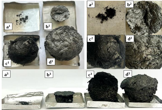
Hình 3.24. Hình ảnh cấu trúc than của EP và các mẫu composit của nó sau khi nung ở 900 °C: EP (a); 10ATH PEI /EP (b); 10APP@PEI/EP (c) và 3ATH PEI /7IFR/EP (d)
